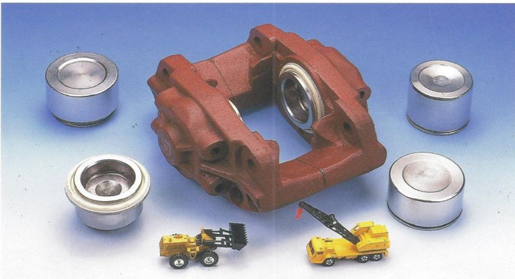
◆ 碟式剎車分泵及活塞
